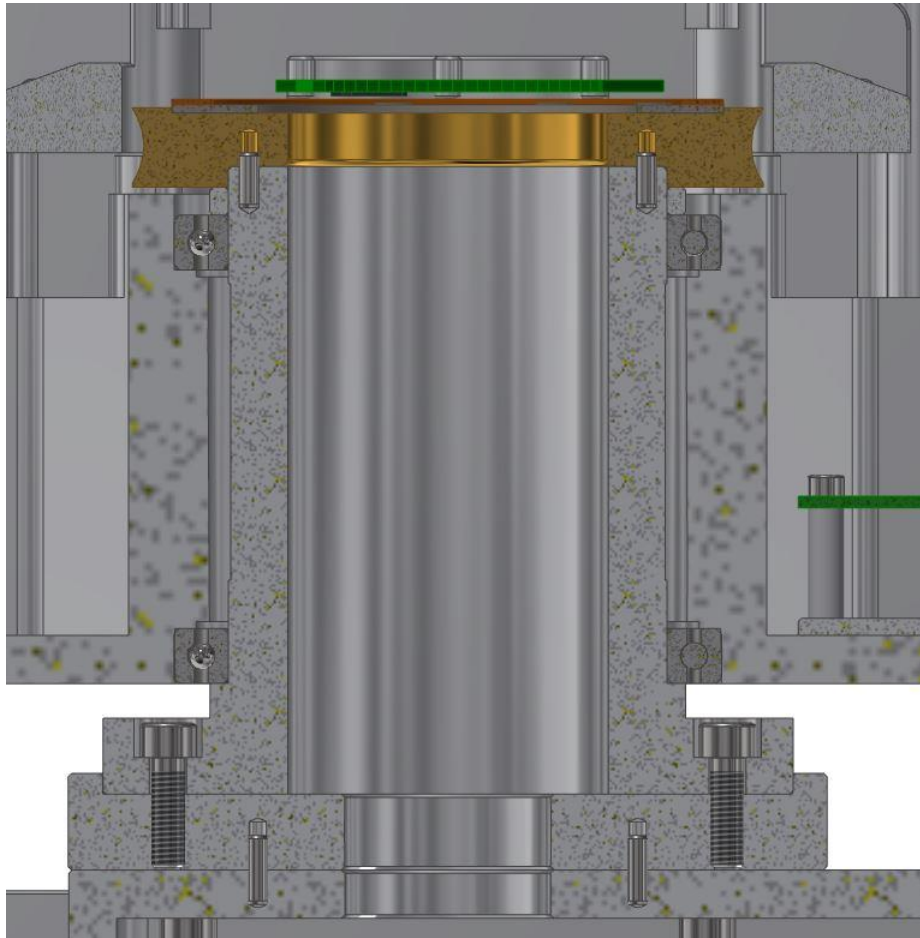
Slika 34. Prikaz presjeka centralne osi rotacije
