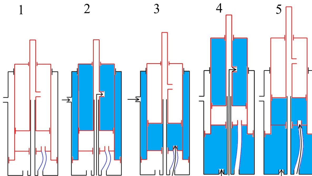
Slika 31. Poprečni presjek i karakteristični radni položaji pneumastkih hvatača (plavo - zrak, crveno - klip hvatača s prstom za hvatanje, crno - kućište hvatača)
