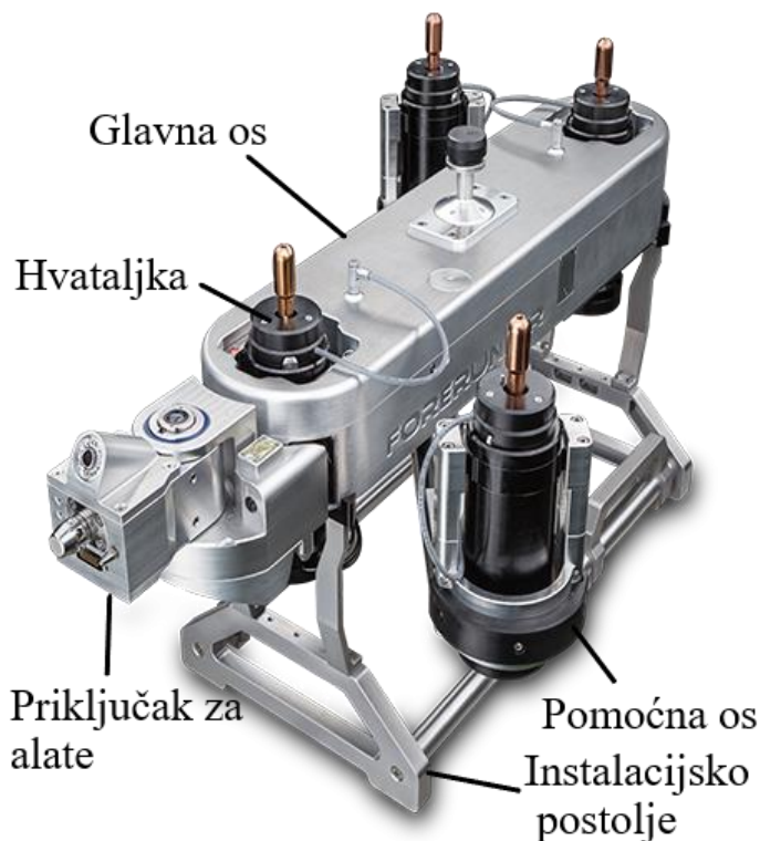
Slika 14. Manipulator Forerunner s osnovnim dijelovima [20]
