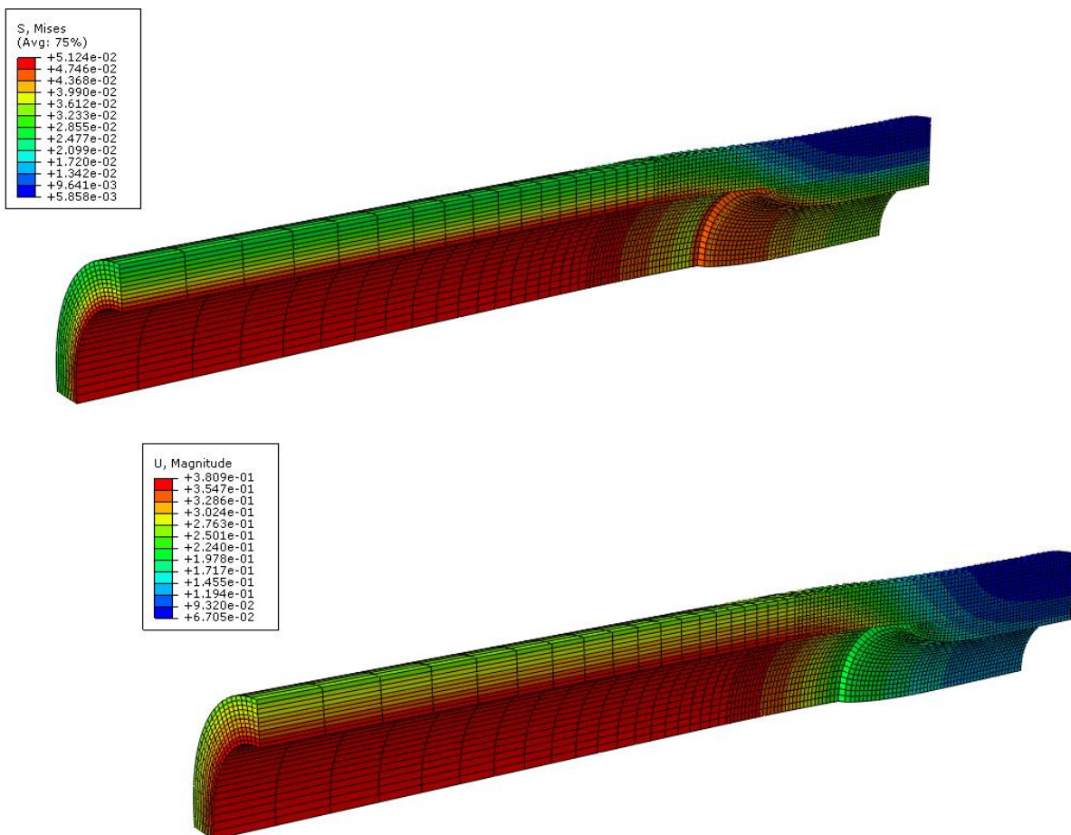
Slika 77. S, Mises naprezanja [N/mm 2 ] i pomaci [mm] na žili s plakom debljine 0,6 mm
