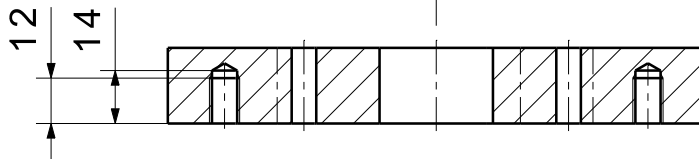
PRESJEK A-A
