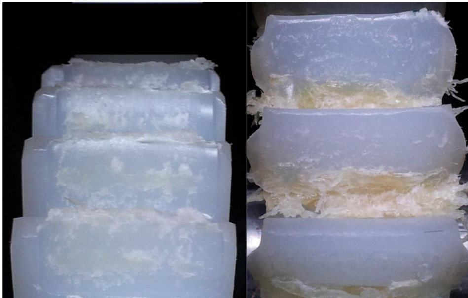
Slika 5.32 Toplinsko zaribavanje polimernih zupčanika gonjenog i pogonskog zupčanika, bok zuba nakon zadovoljavanja radnog uvjeta
