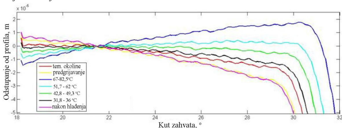
Slika 3.8 Odstupanje profila boka zuba pri različitim temperaturama [69]
