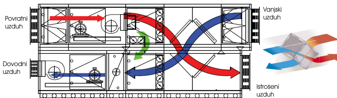
Slika 26. Klima komora sa pločastim rekuperatorom (GEA ECOPLAT)
