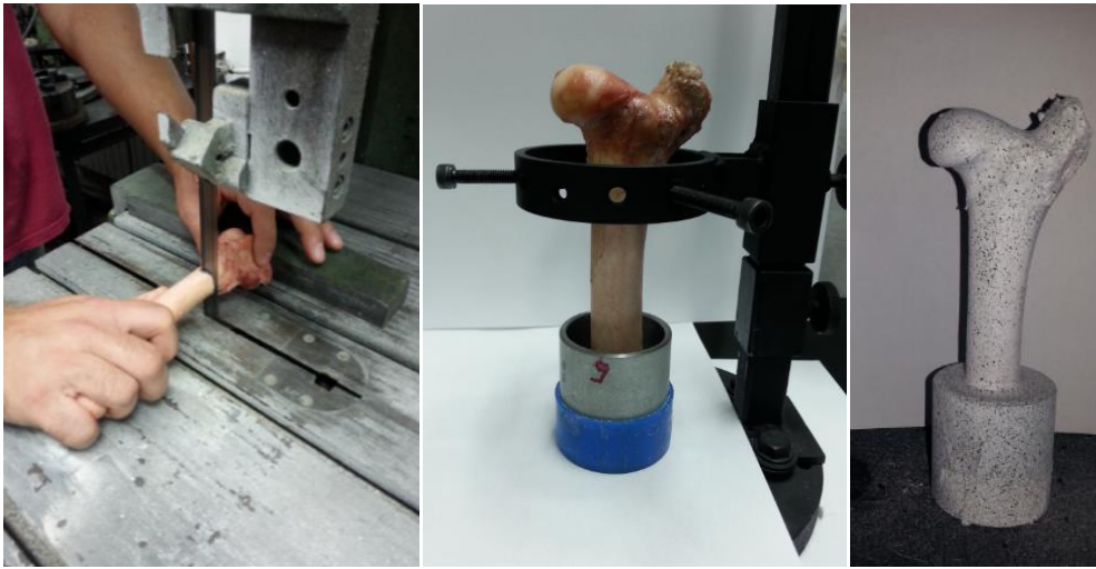
Slika 35. Priprema ovčjeg femura za mehaničko ispitivanje
