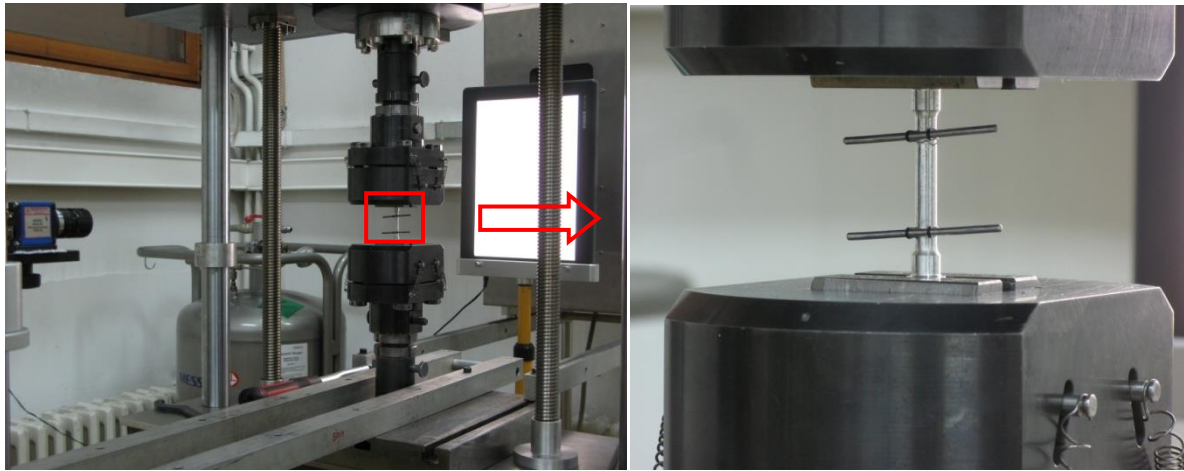
Slika 9. Mjerenje videoekstenzometrom
