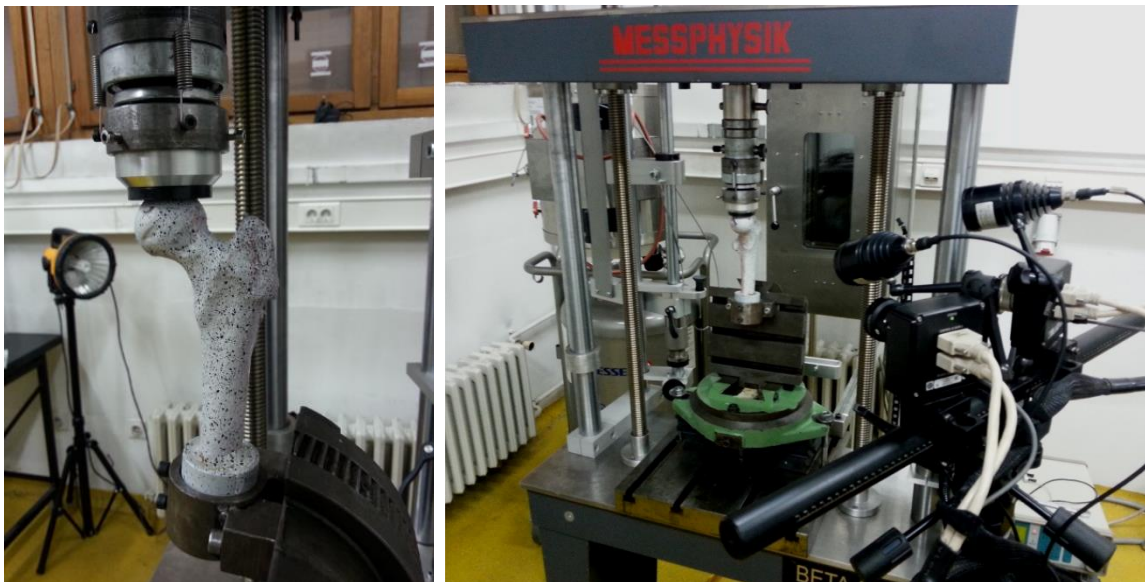
Slika 39. Ispitni uzorak kadaveričnog femura pripremljen za mehaničko ispitivanje
