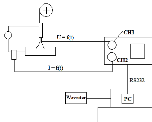
Slika 4.12 Shema spajanja mjerne opreme [20]
