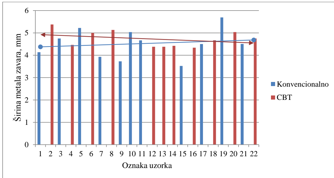
Slika 5.19 Grafički prikaz promjene nadvišenja metala zavara ovisno o variranim parametrima za konvencionalno MAG i CBT MAG zavarivanje
