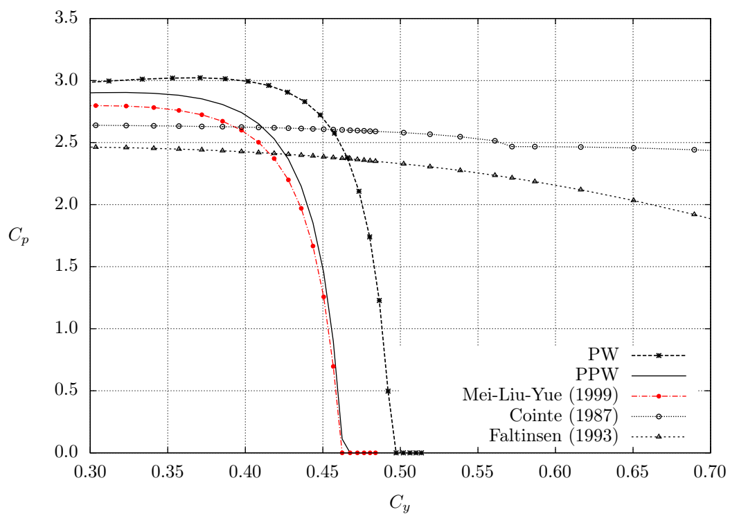
Slika 4.19: Usporedba prostorne raspodjele tlaka za klin nagiba 45^\circ
