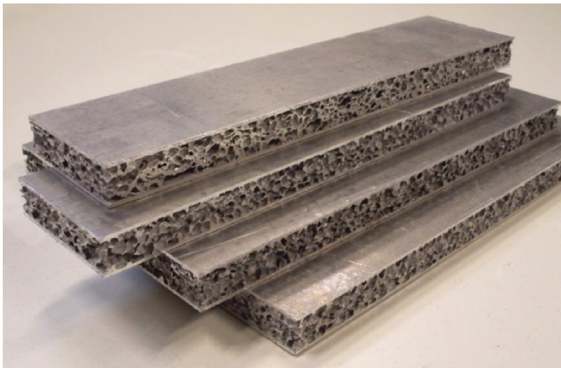
Slika 2.13. Aluminijski sendvič paneli s aluminijskom pjenom kao jezgrom
