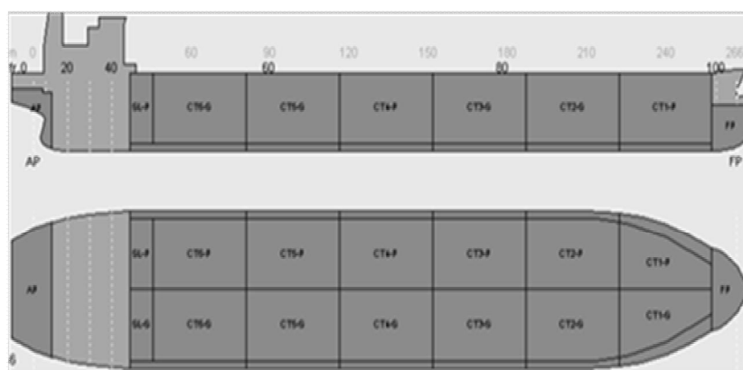
Slika 5.1. Opći plan Aframax tankera
