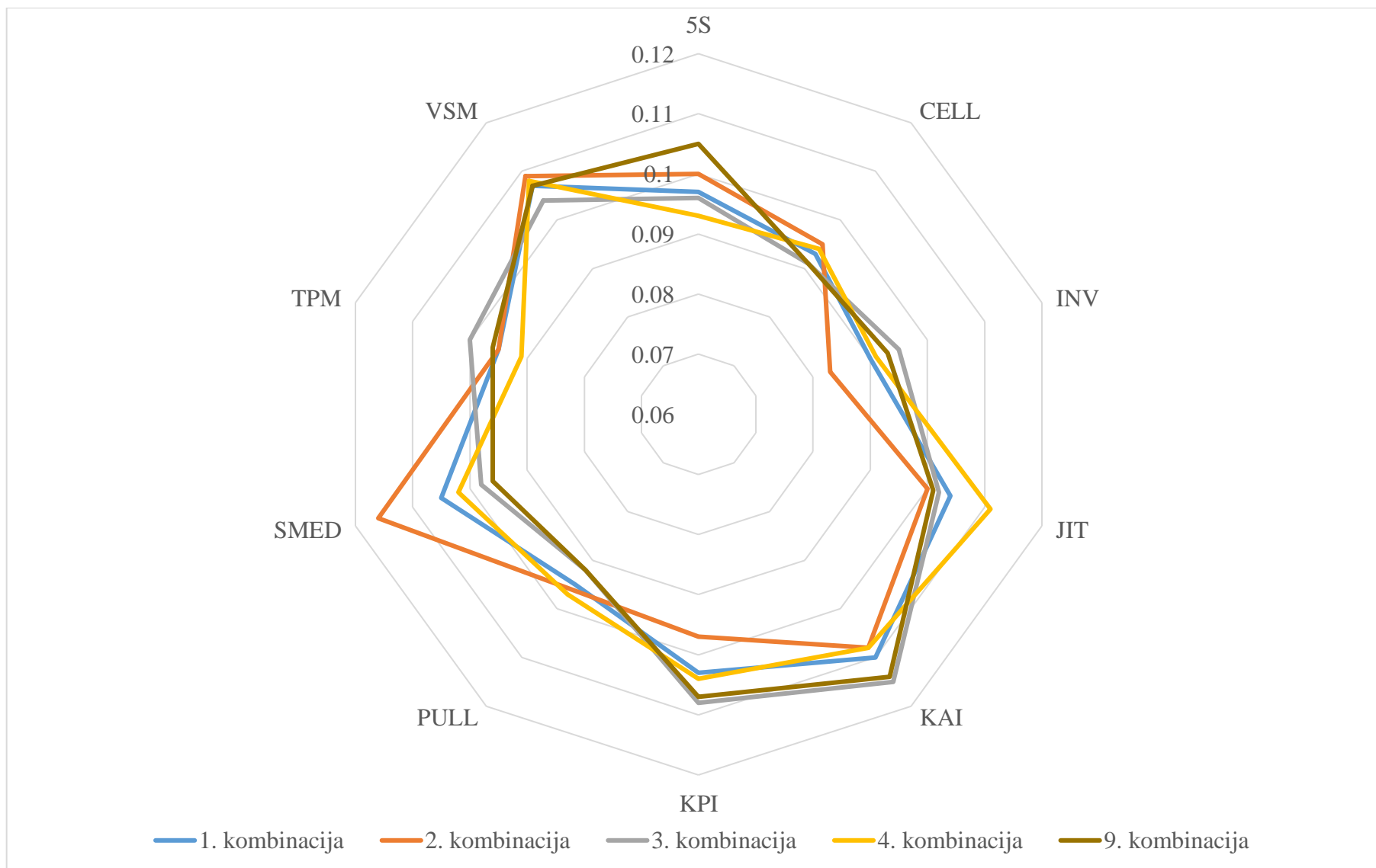
Slika 5.29 – Usporedba vrijednosti vektora prioriteta alternativa 1., 2., 3., 4. i 9. kombinacije
