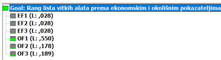
Slika 5.17 – Vektor prioriteta kriterija za 6. kombinaciju
