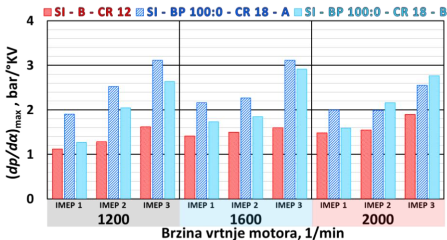
Slika 4.22. Usporedba najvećih srednjih vrijednosti brzina porasta tlaka u cilindru motora
