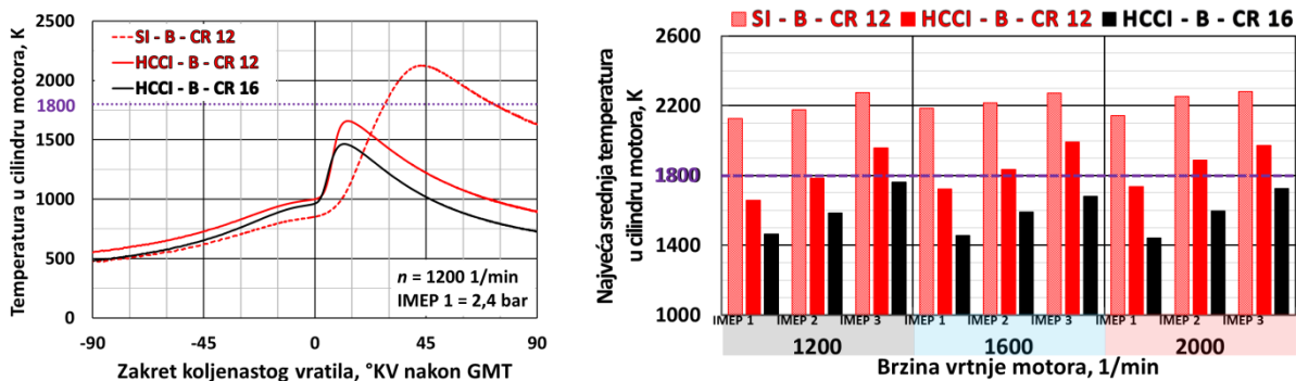
Slika 4.10. Profili srednje temperature u cilindru motora (lijevo) i usporedba najvećih srednjih vrijednosti temperatura u cilindru motora (desno)
