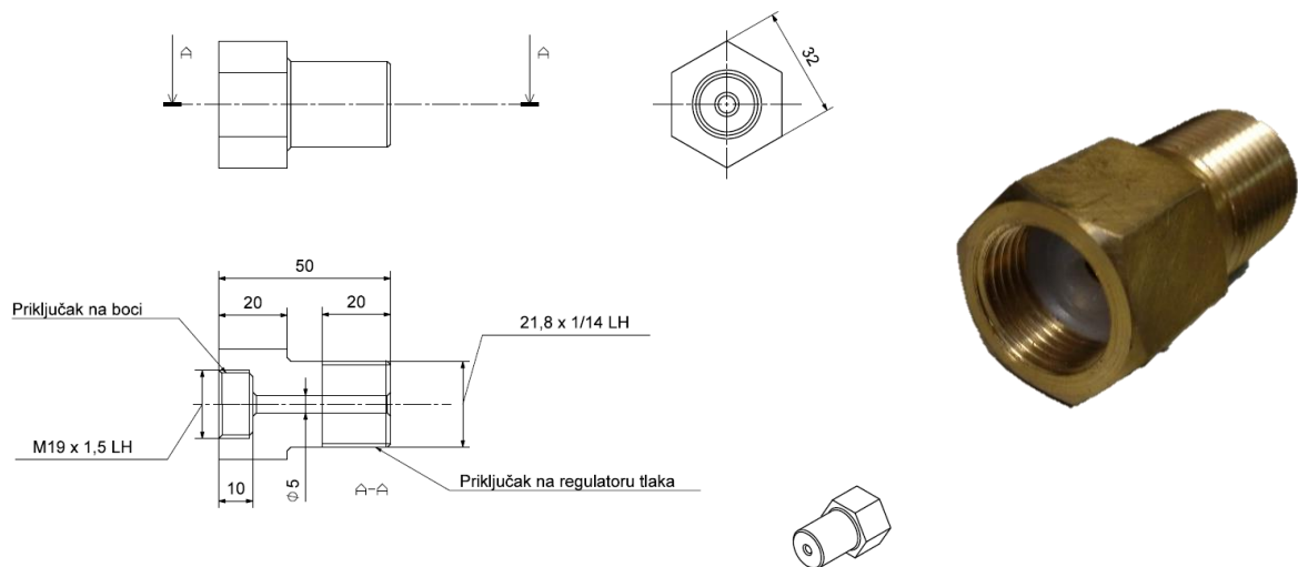
Slika 2.42. Adapter za boce s plinovitim gorivom na regulator tlaka (lijevo) i fotografija izrađenog adaptera (desno)
