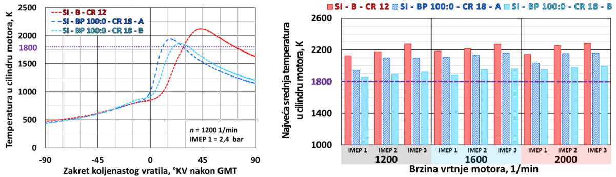
Slika 4.23. Prikaz profila temperature u cilindru motora (lijevo)
