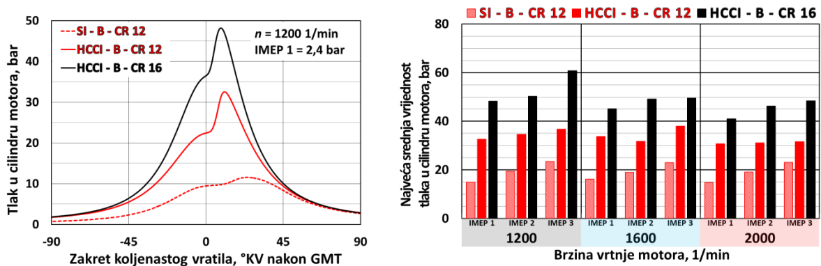
Slika 4.6. Prikaz profila tlaka u cilindru motora (lijevo) i usporedba najvećih srednjih vrijednosti tlaka u cilindru motora (desno)
