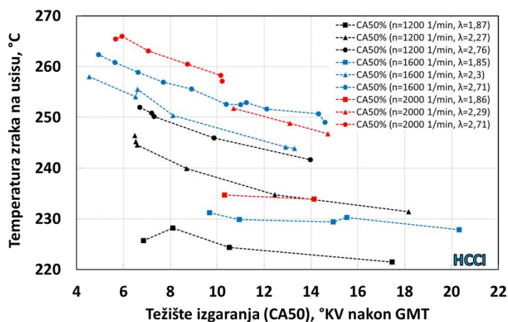
Slika 3.6. Kontrola izgaranja u HCCI načinu rada.
