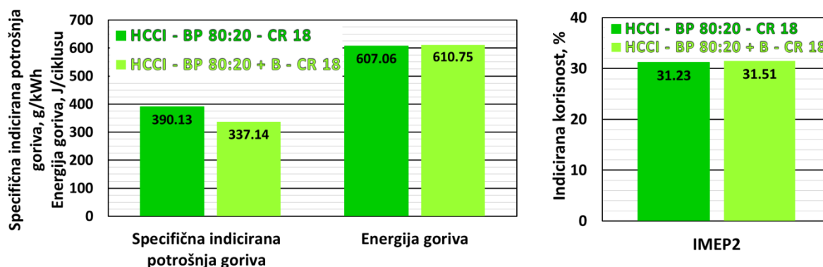
Slika 4.82. Usporedba specifične indicirane potrošnje goriva i energije dovedene gorivom po ciklusu (lijevo) i indicirana korisnost motora (desno)
