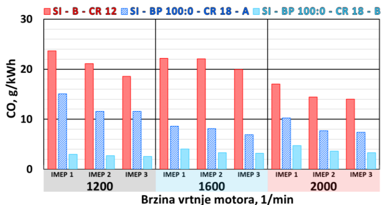
Slika 4.29. Usporedba emisije CO
