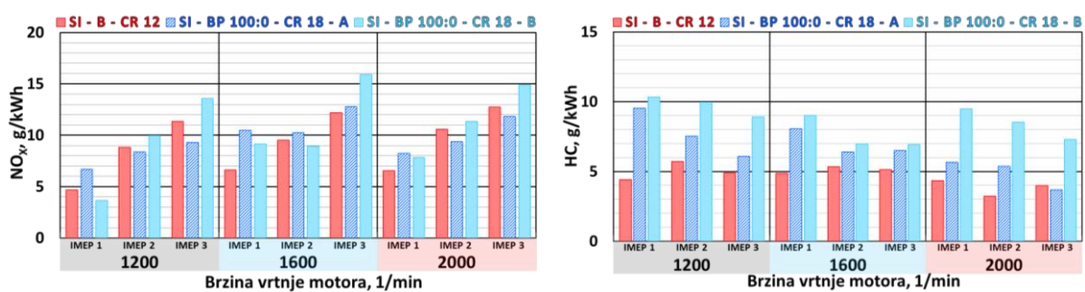
Slika 4.28. Usporedba emisije NO_x (lijevo) i HC (desno)
