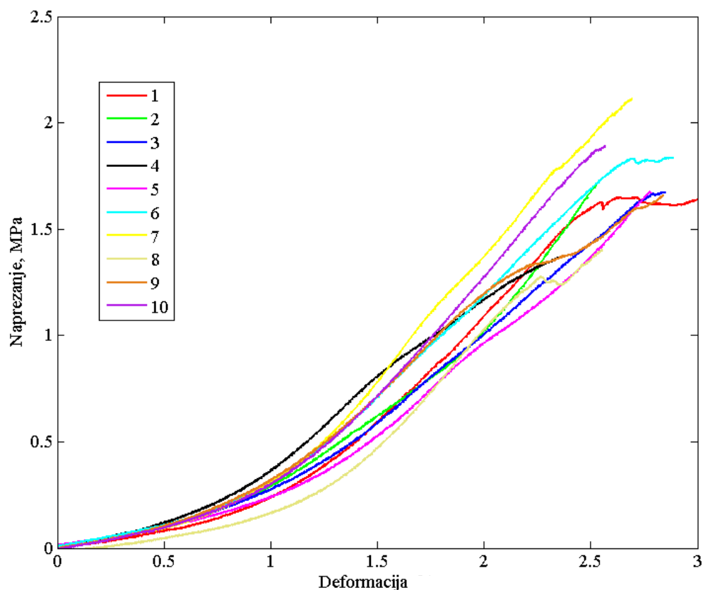
Slika 90. Dijagram deformacija-naprezanje svježih poprečnih uzoraka aorte za pohranu od devet mjeseci
