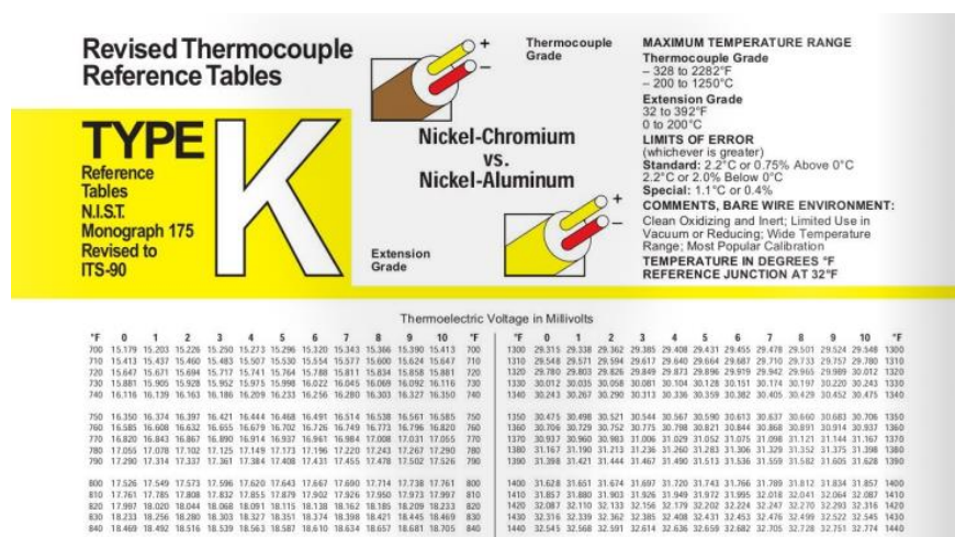
Slika 2.36. Dio tabličnog prikaza vrijednosti termopara tipa K i modul NI 9213 za očitavanje temperature [70]
