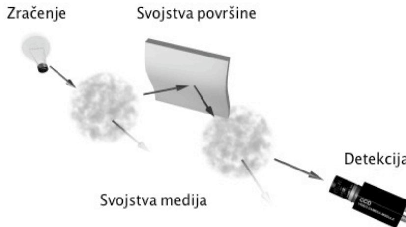
Slika 2.7 Lanac zračenja [2]
