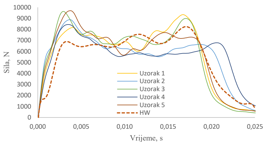
Slika 40. Krivulje sile udara u apsorbirajućem profilu pri v_0 = 7 \text{ ms}^{-1}
