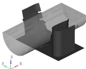
Slika 49. Deformirani oblik u trenutku maksimalne intruzije udarača ( t = 20,6 \text{ ms} ) u apsorber „otvorenog“ profila pri v_0 = 10 \text{ ms}^{-1}
