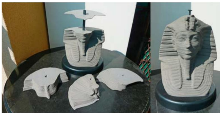
Slika 1. Princip aditivne proizvodnje [2]
