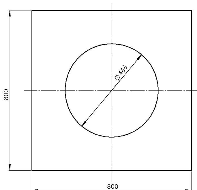
Slika 23. Dimenzije ploče
