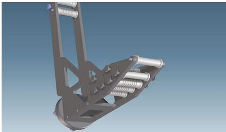
Slika 19. Naprava za dodavanje vlakana s valjcima [16]
