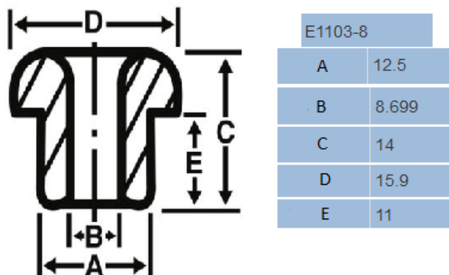
Slika 26. Keramička vodilica [17]
