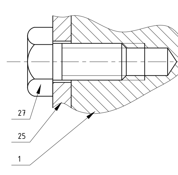
Presjek D-D (M 2:1) Prikaz spoja poklopca ležaja
