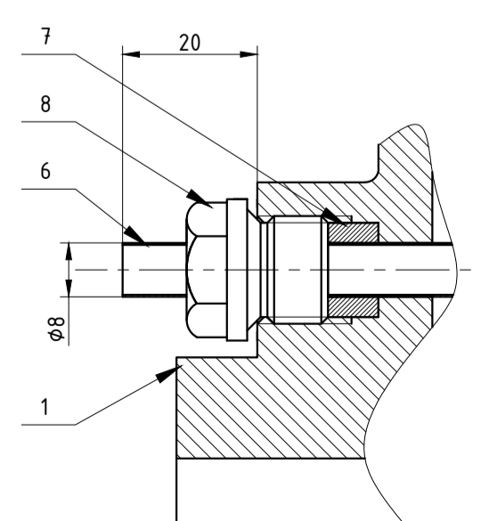
Presjek B-B (M 1:1) Prikaz spoja cijevne zmije
