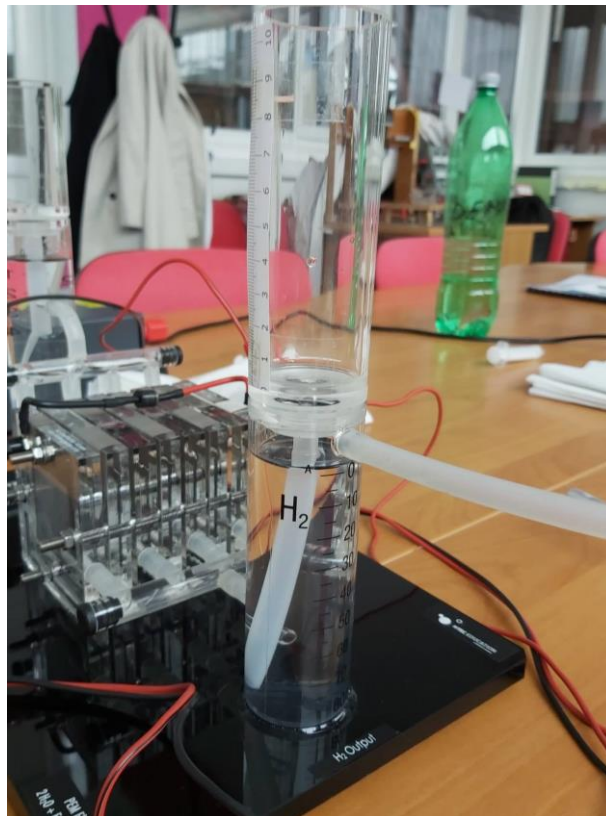
Slika 5.7 Spremnik vodika
