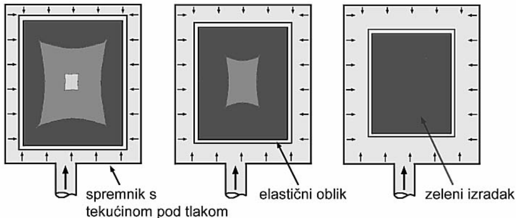
Slika 12 Izostatičko prešanje s područjima različitog zgušnjavanja [1]
