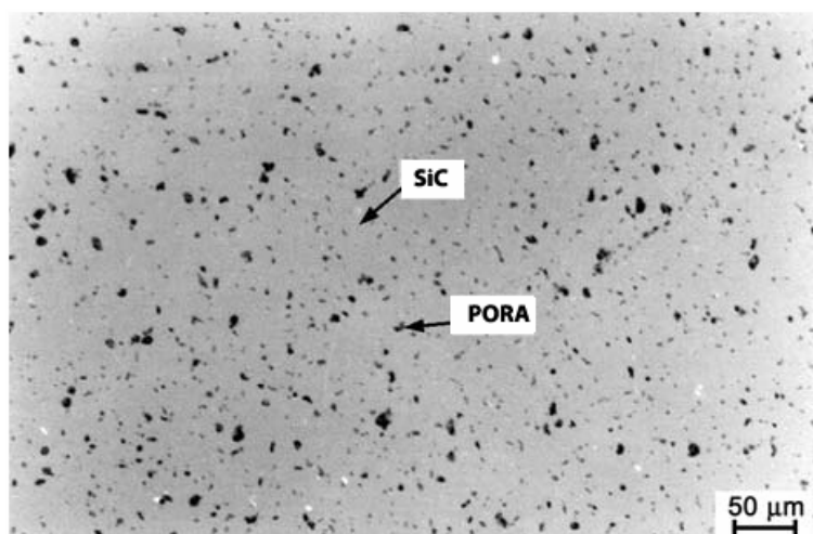
Slika 4 Mikrostruktura SSIC [1]
