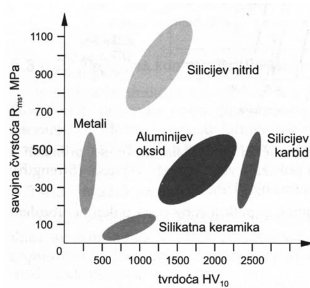
Slika 16 Područja vrijednosti tvrdoća i savojne čvrstoće [1]
