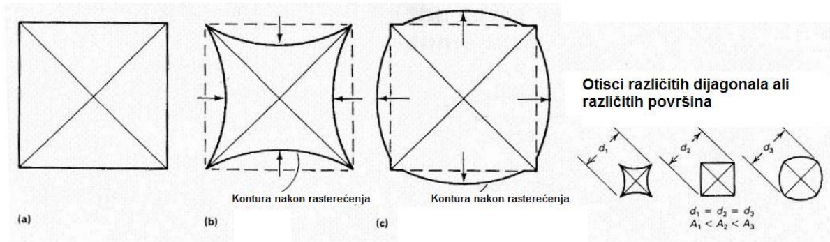
Slika 21 Prikaz anomalija za otiske kod Vickersove metode [11]
