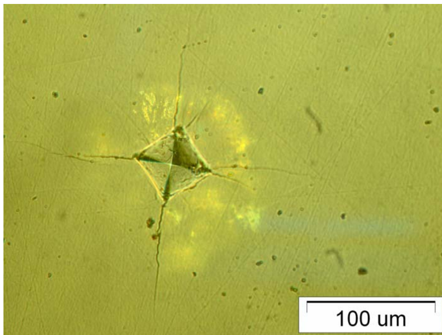
Slika 30 Otisak dijamentne piramide nakon mjerenja tvrdoće metodom HV5
