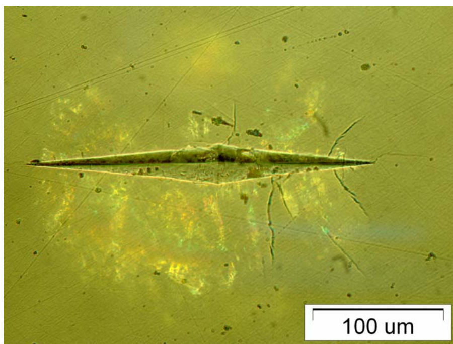
Slika 40 Otisak dijamentne piramide nakon mjerenja tvrdoće metodom HK10
