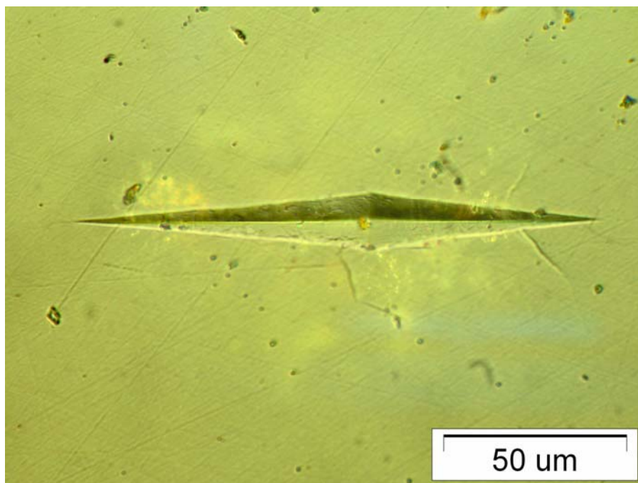
Slika 38 Otisak dijamentne piramide nakon mjerenja tvrdoće metodom HK3
