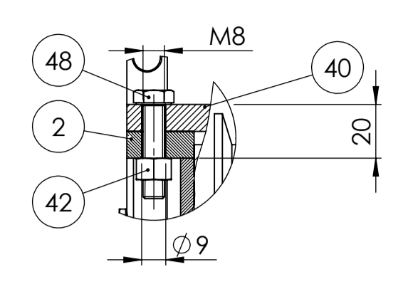
Detalj D 1:1
