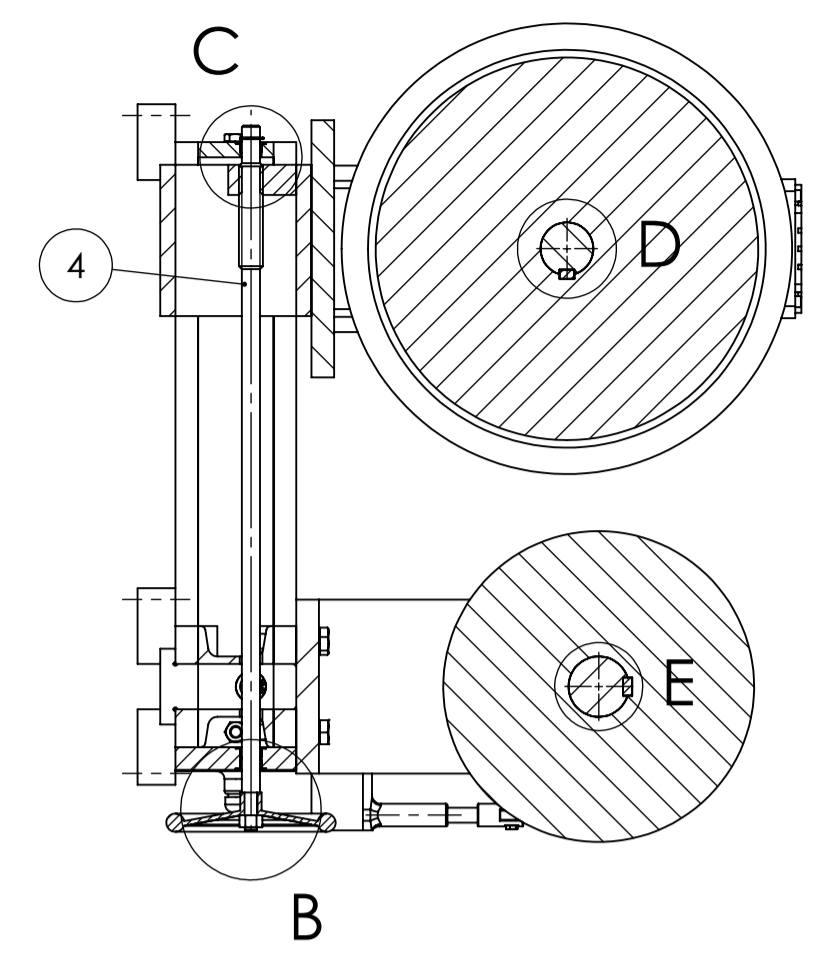
Presjek C-C
