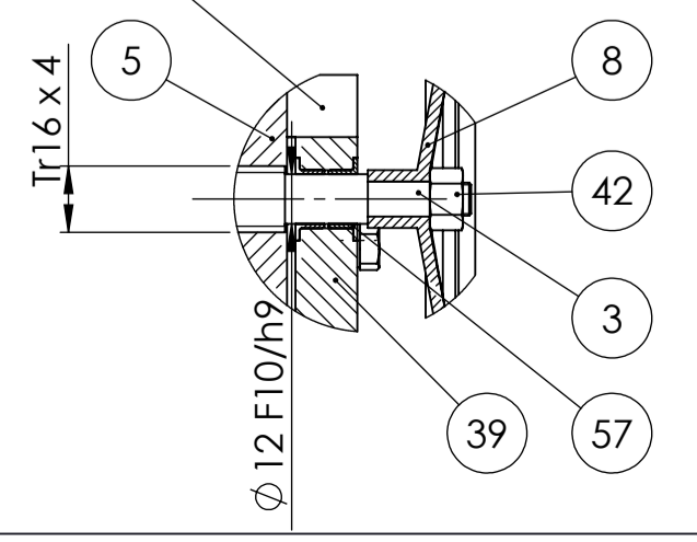
Detalj R 1:2
