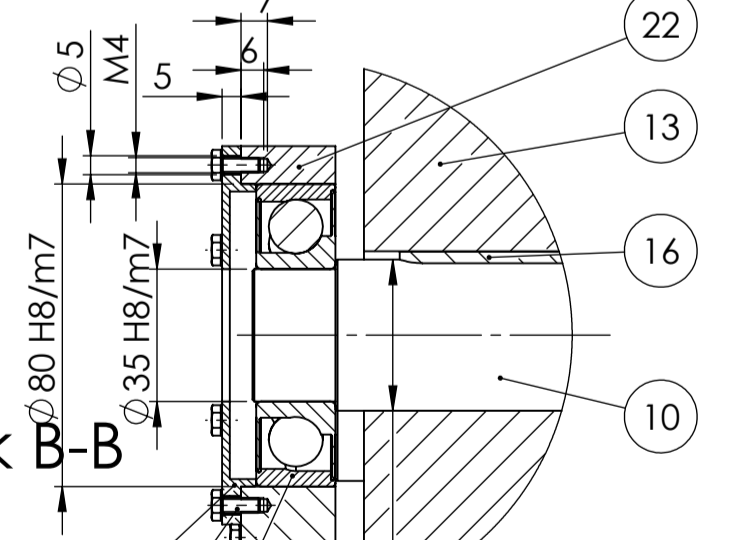
Detalj M 1:2
