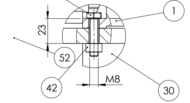
Detalj L 1:2
