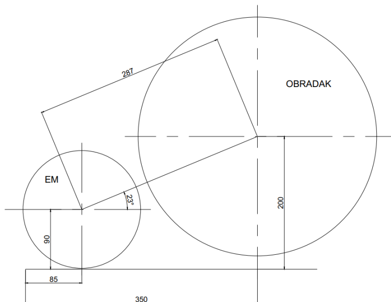
Slika 16. Osni razmak
