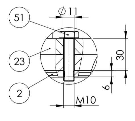
Detalj K 1:2
