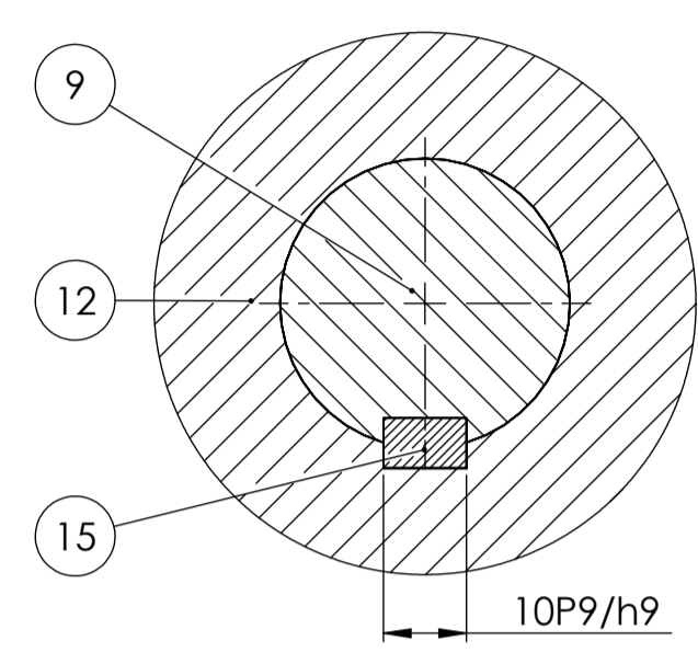
Detalj I 1:2
