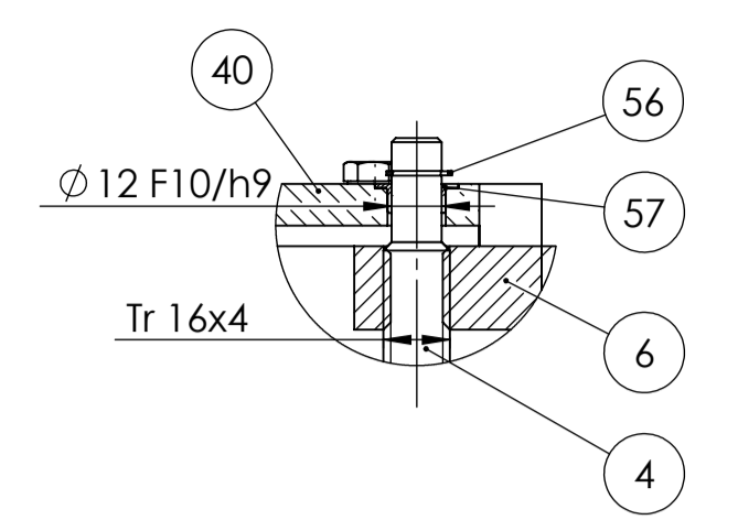
Detalj C 1:2
