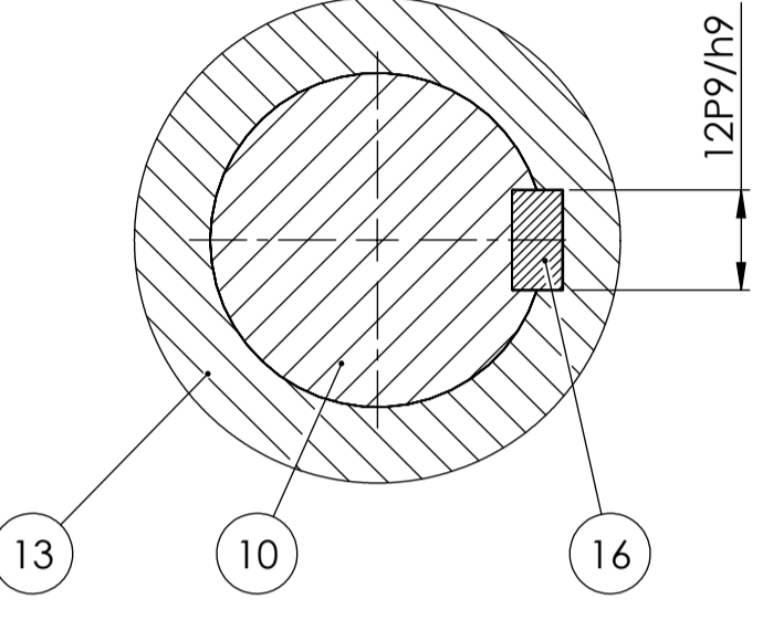
Detalj E 1:1
