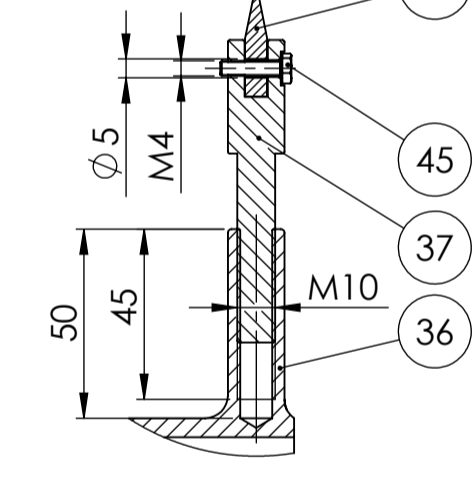
Detalj N 1:1
