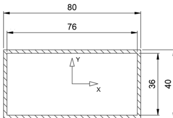
Slika 25. Presjek stupa
