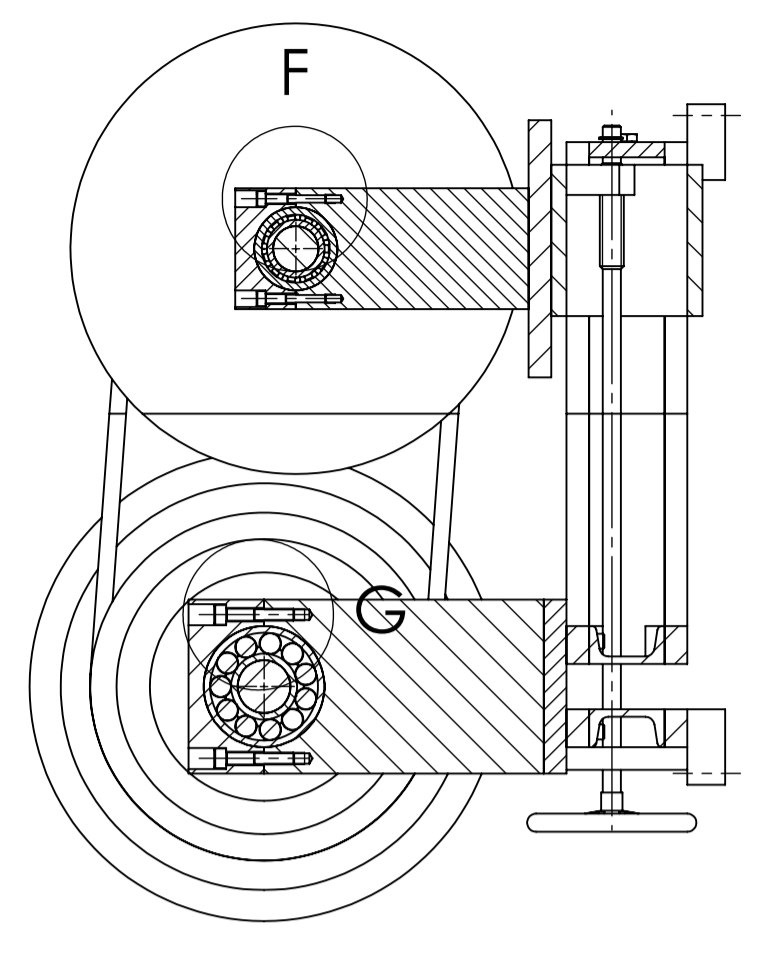
Presjek D-D
