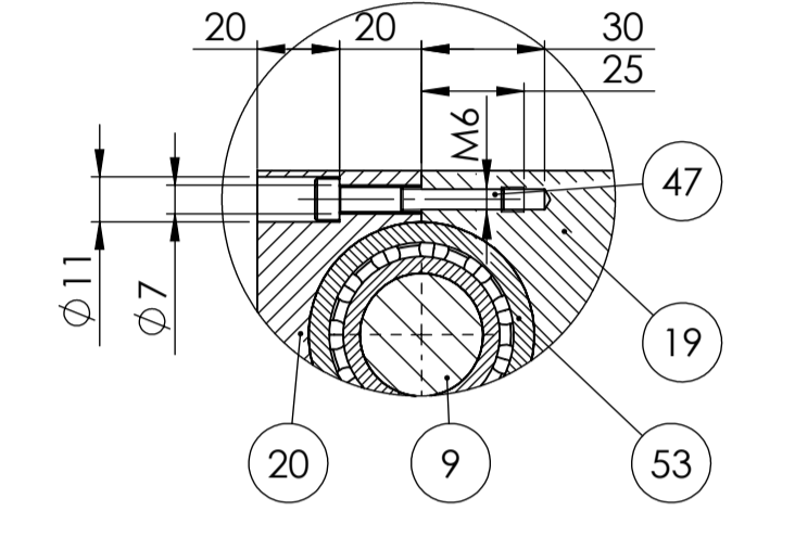
Detalj F 1:2
