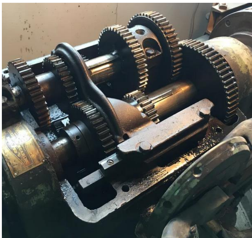
Slika 8. Zupčanički prijenosnik na tokarskom stroju
