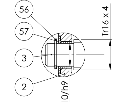
Detalj N 1:1
