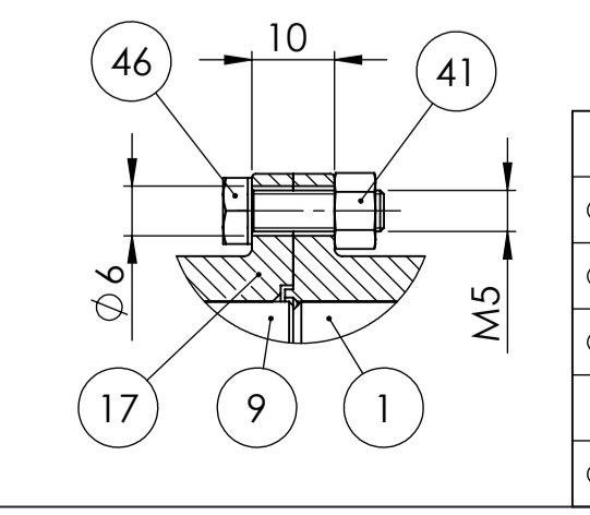
Detalj T 1:1
