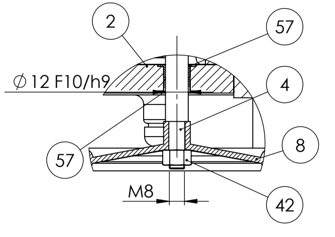
Detalj E 1:1
