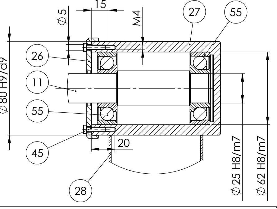
Detalj P 1:2
