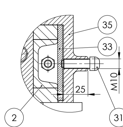
Detalj L 1:2
