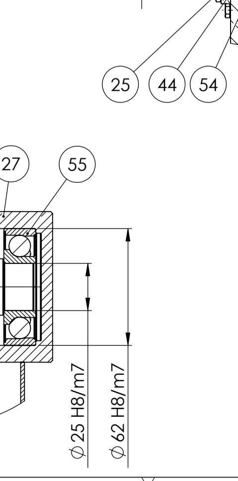
Presjek B-B
