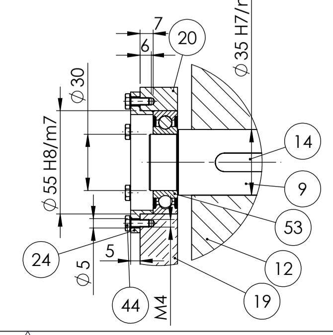
Detalj S 1:2
