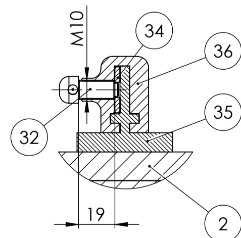
Detalj O 1:2
