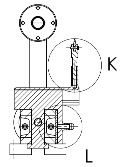
Presjek E-E
