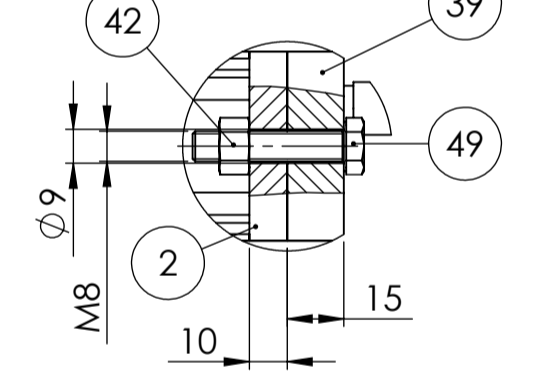
Detalj M 1:2
