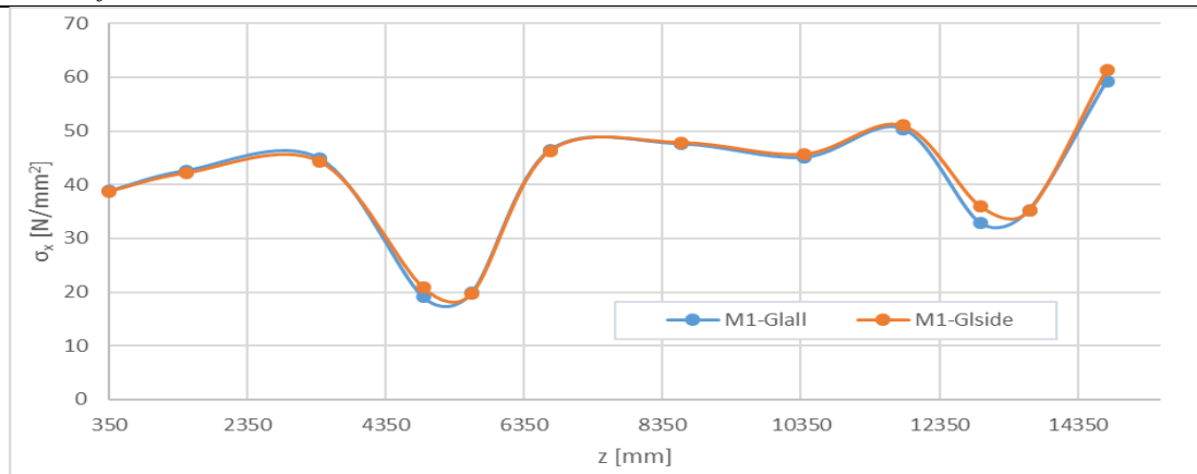
Slika 33 Raspodjela \sigma_x naprezanja modela M1 po širini palube šest
