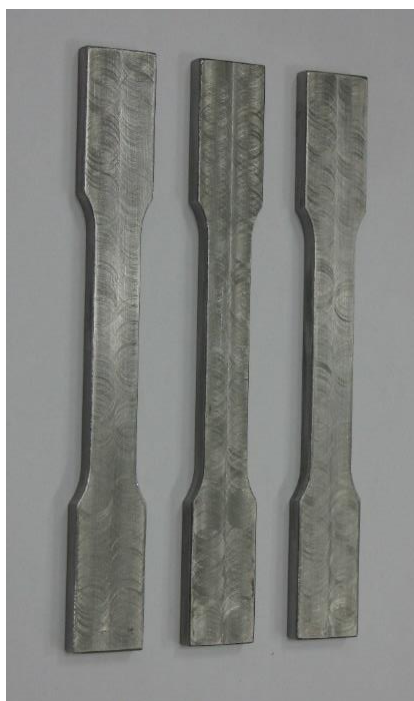
Slika 18. Ispitni uzorci a) iz konstrukcijskog čelika i b) iz nodularnog lijeva
