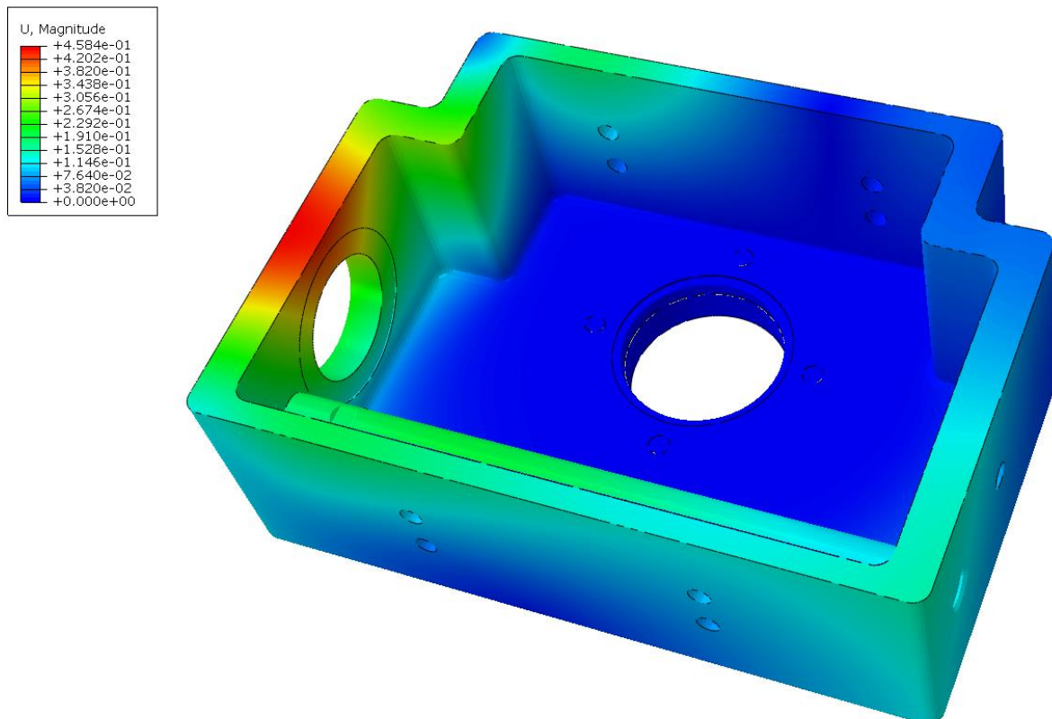
Slika 31. Pomaci kod prve lijevane izvedbe kućišta
