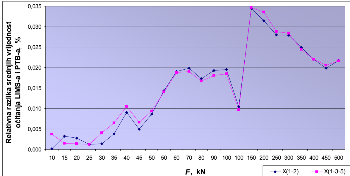
Slika 41 – Usporedni prikaz relativnih razlika srednjih vrijednosti očitavanja bez i sa rotacijom između PTB-a i LIMS-a za čitavo mjesto područje od 10 kN do 500 kN
