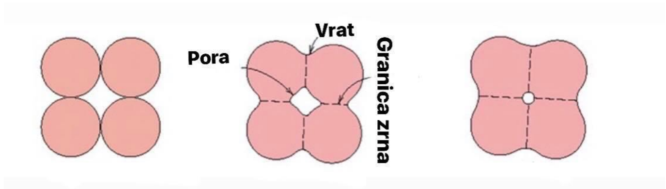
Slika 4. Zgušnjavanje i spajanje kuglica praha sinteriranjem [6]
