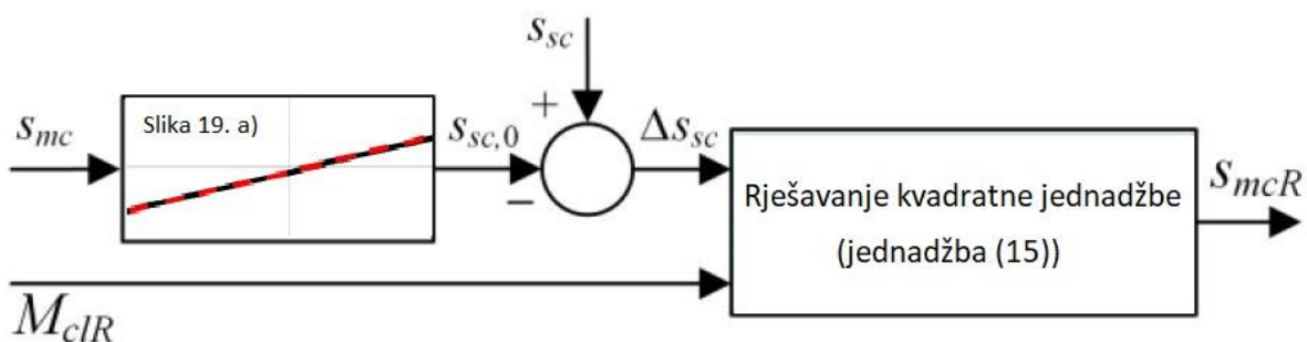
Slika 20. Blok dijagram upravljačke strategije [1]
