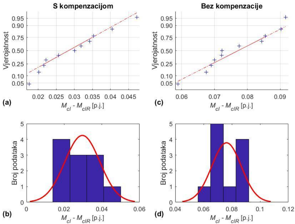
Slika 35. Raspodjela reziduala M_{cl} - M_{clR} s kompenzacijom ((a) i (b)) i bez kompenzacije ((c) i (d)) termalnih efekata za raspon temperatura spojke 0.492 – 0.515 p.j.
