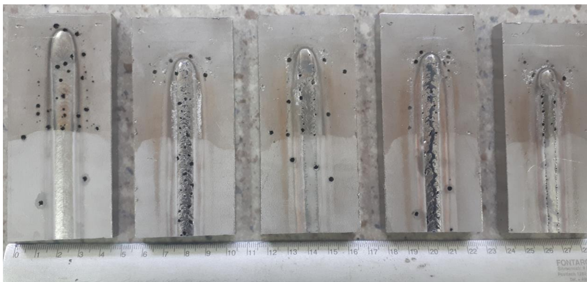
Slika 40. Izgled očišćenih površina uzoraka nakon 48 h u otopini
