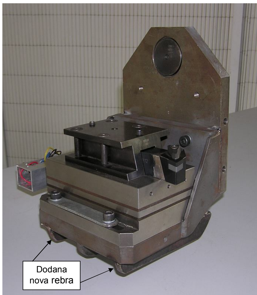
Slika 59. Poboljšana naprava za prihvat mjerača sila
