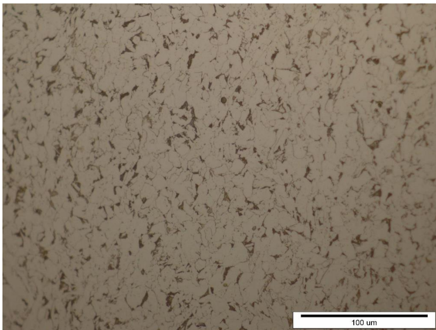
Slika 31. Mikrostruktura osnovnog materijala okomito na smjer valjanja nakon nagrizanja snimljena pri povećanju od 500×
