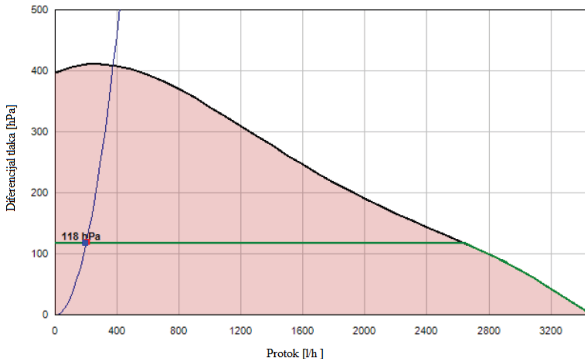
Slika 30. Krivulja crpke
