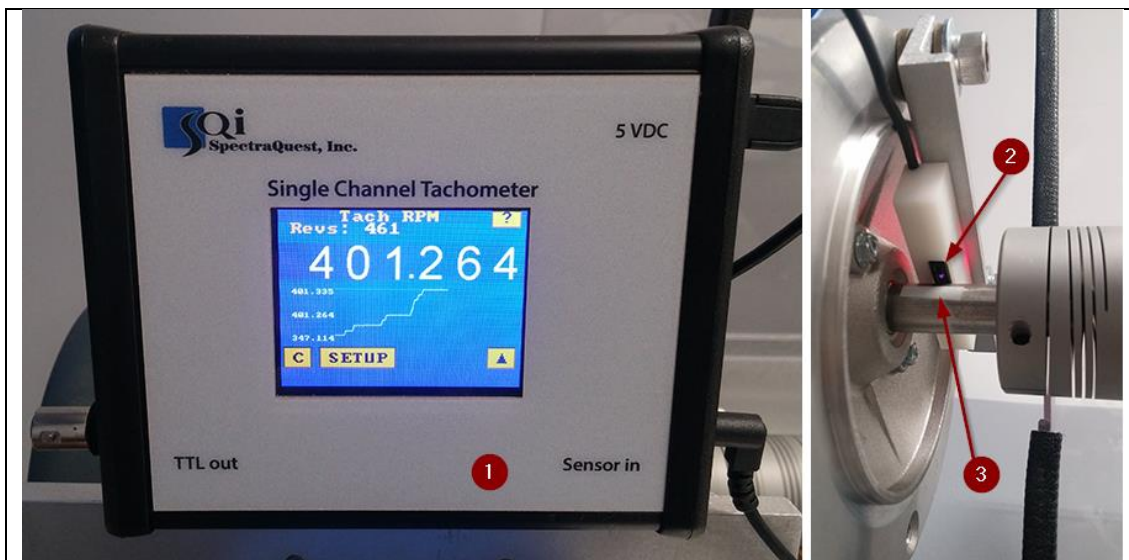
1. Ekran s prikazom učestalosti vrtnje, 2. Optički referentni senzor, 3. Reflektirajuća traka
