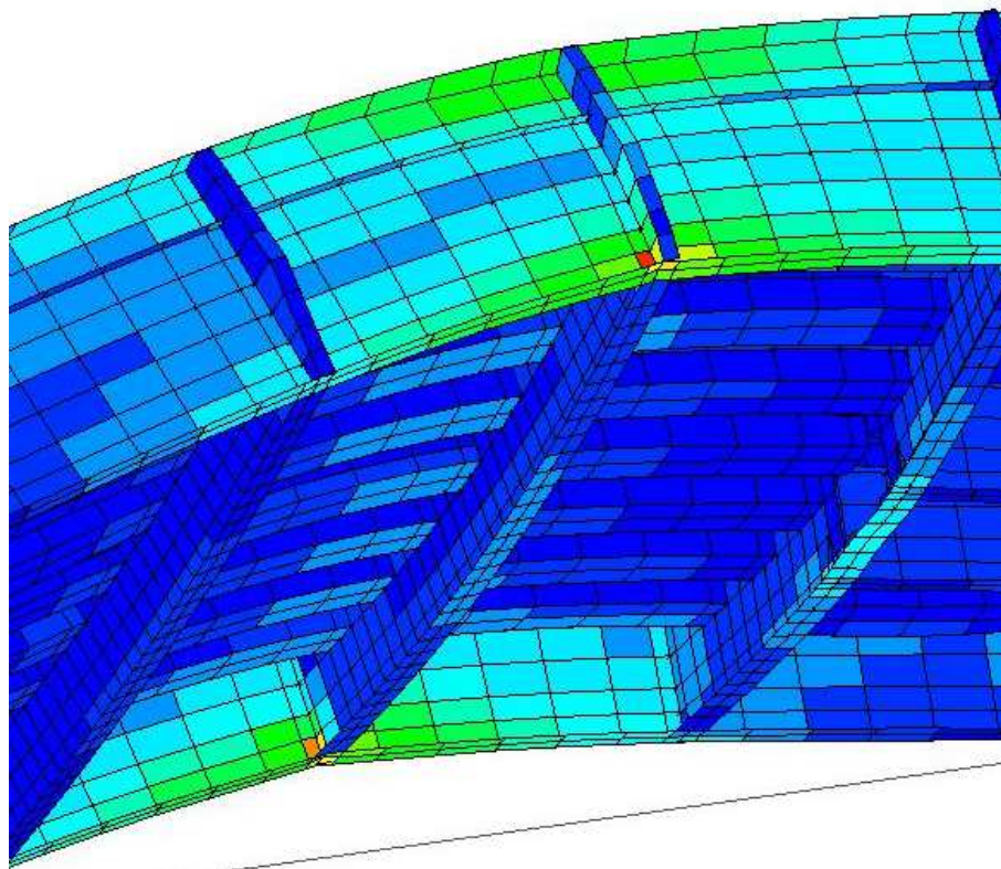
Slika 29. Najveća von Mises naprežanja LCH-2
