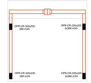
Detalji odsisnog kanala OP dvorane
