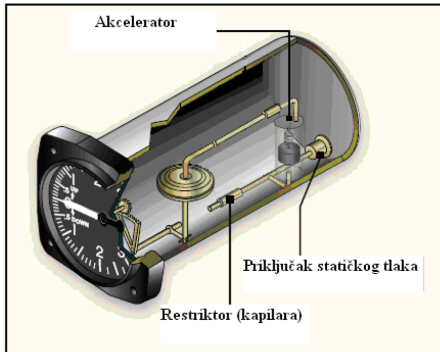
Slika 2.11. Shematski prikaz instantanog variometra [4].
