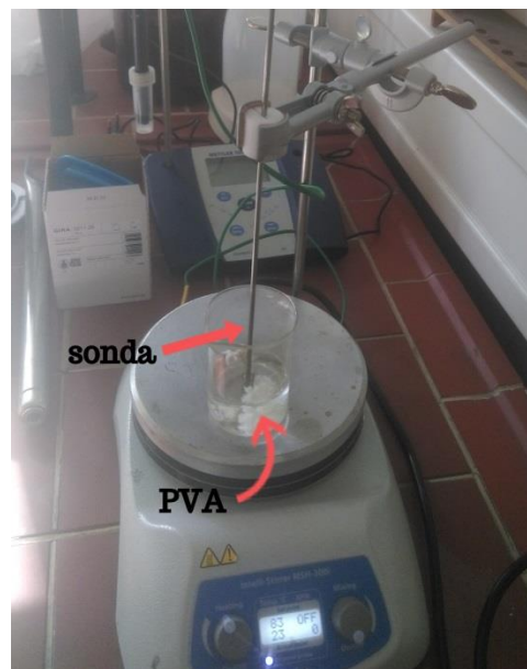
Slika 20. Otapanje PVA
