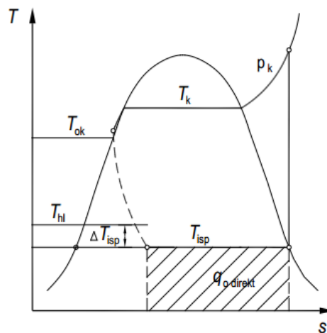
Slika 1. Ljevokretni kružni proces [2]
