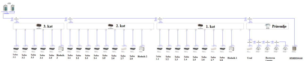
Slika 45. Shema cijevnog razvoda VJ 3 [6]
