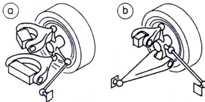
Slika 2.9 Neovisni ovjes s dvije poprečne vodilice
