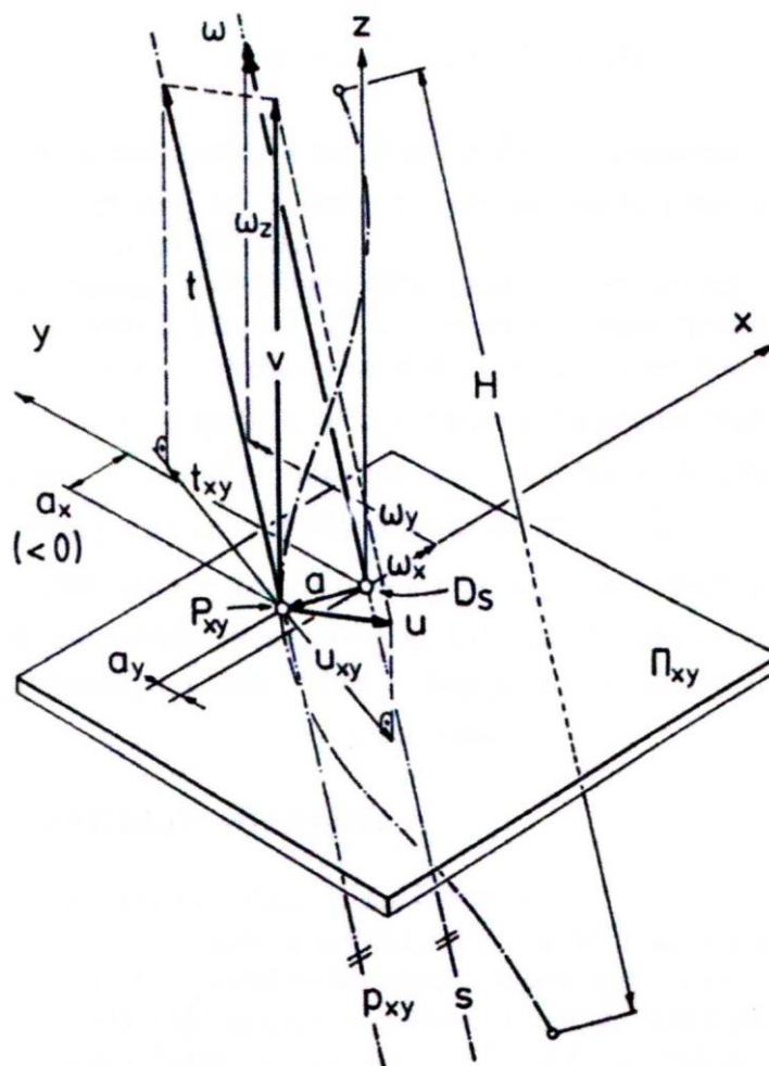
Slika 3.4 Prikaz vijčane osi s i trenutnog pola P_{xy} u ravnini \Pi_{xy}
