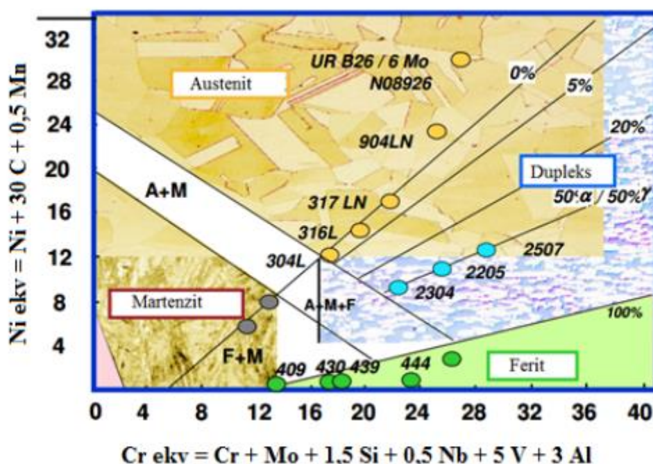
Slika 4. Schaeffler-ov dijagram [10]
