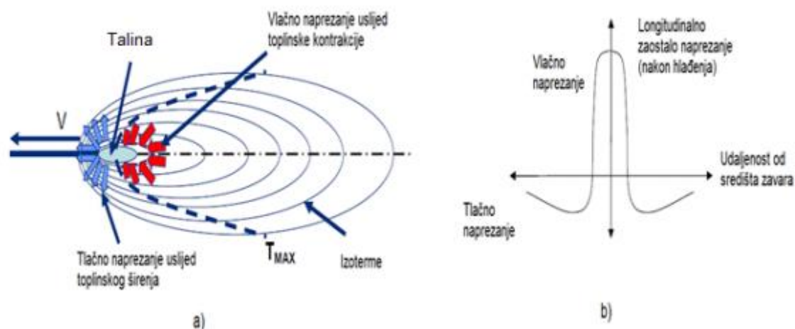
Slika 23. Napreznja u zoni zava: a) Toplinsko napreznje tijekom zavarivanja; b) Longitudinalno zaostalo napreznje nakon hlađenja [42]
