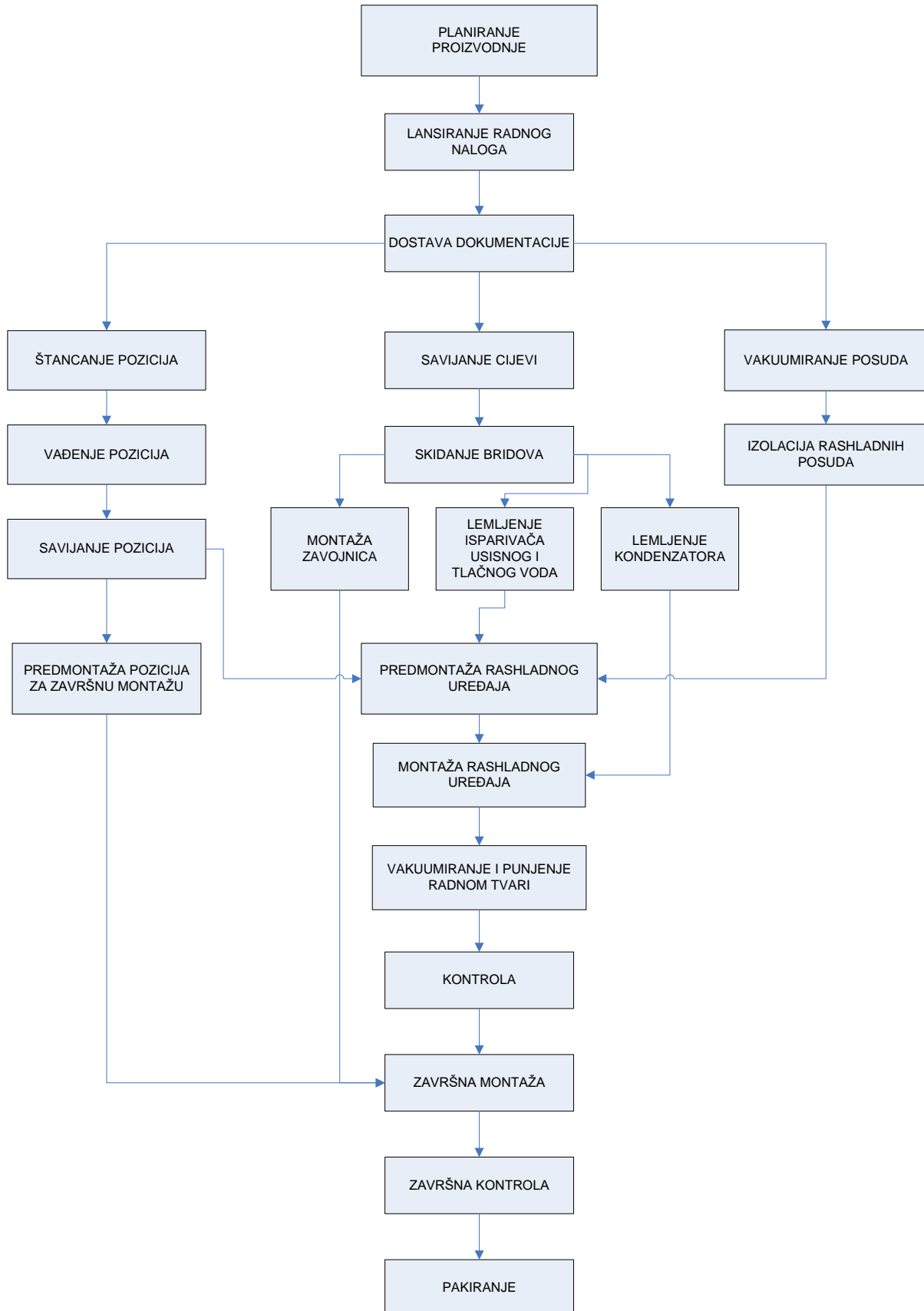
Slika 13. Dijagram toka proizvodnog procesa [10]
