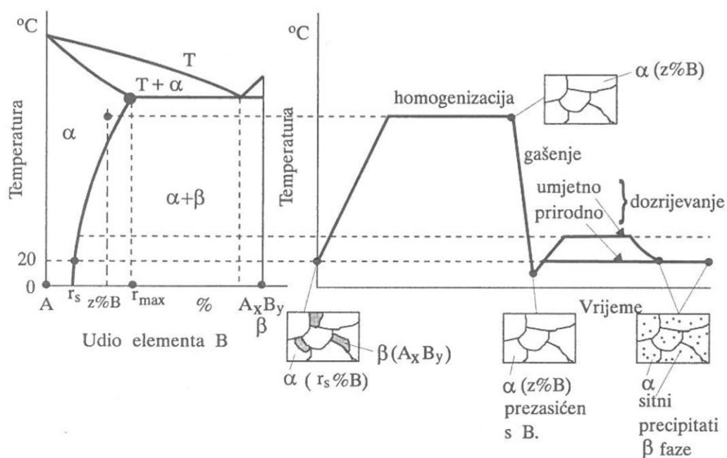
Slika 1. Postupak precipitacijskoga očvrnuća [1]
