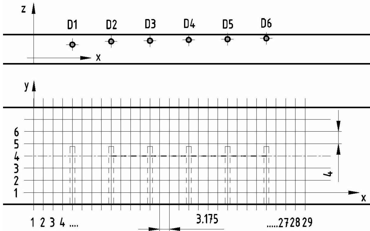
Slika 4.3. Raster na površini etalona Test Bar-a
