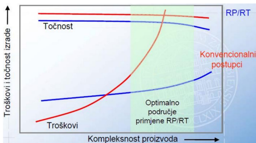
Slika 7. Usporedba aditivnih tehnologija s konvencionalnim metodama [13]
