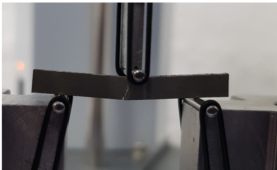
Slika 58. Izgled loma šuplje epruvete
