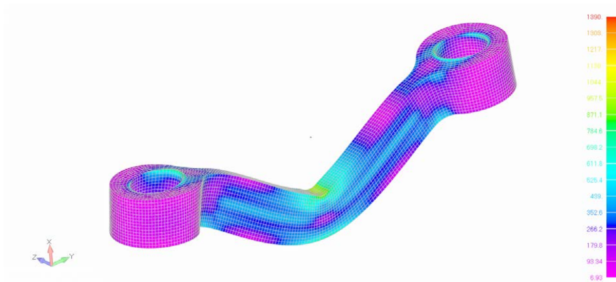
Slika 43. Naprezanja koja se javljaju u modelu
