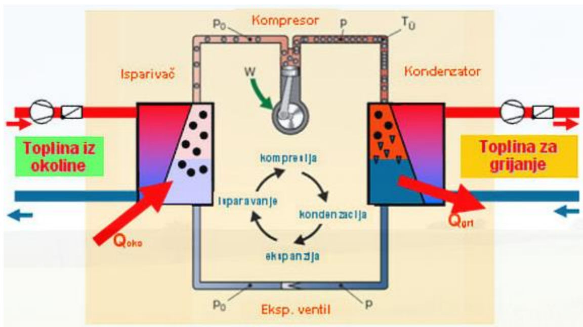
Slika 3. Prikaz načina prijenosa topline i cirkulacije radne tvari kroz dizalicu topline [4]
