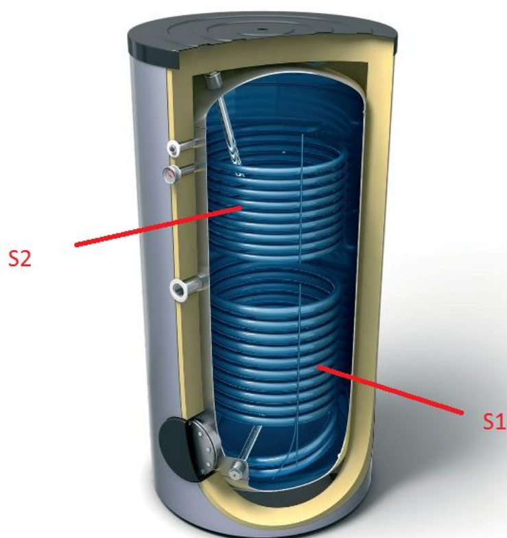
Slika 24. Bosch akumulacijski spremnik AS DUO 1000[14]
