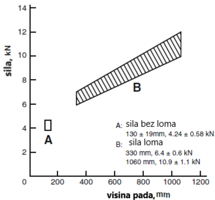
Slika 7. Tolerancija lubanje na udarac s obzirom na silu [1]
