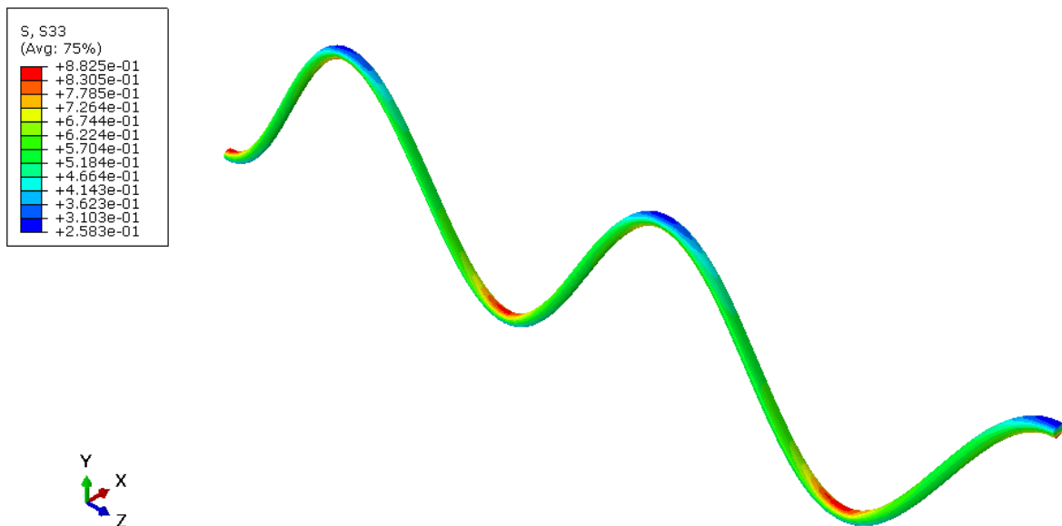
Slika 22. Raspodjela Cauchyevog naprezanja na polovini zavojnice koncepta 1
