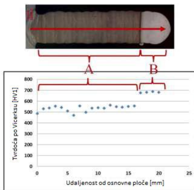
Slika 19. Tvrdoća po presjeku [15]
