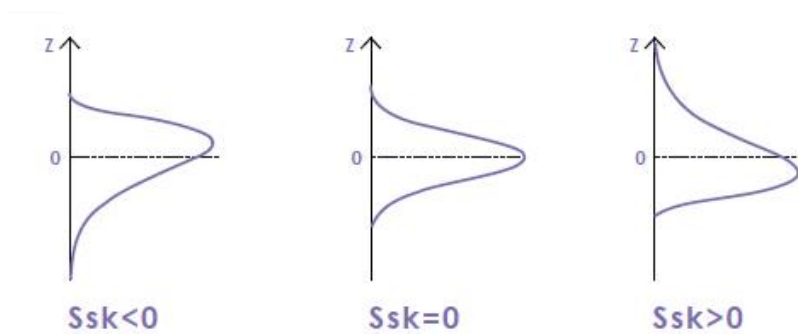
Slika 10. Koeficijent asimetrije površine [12]
