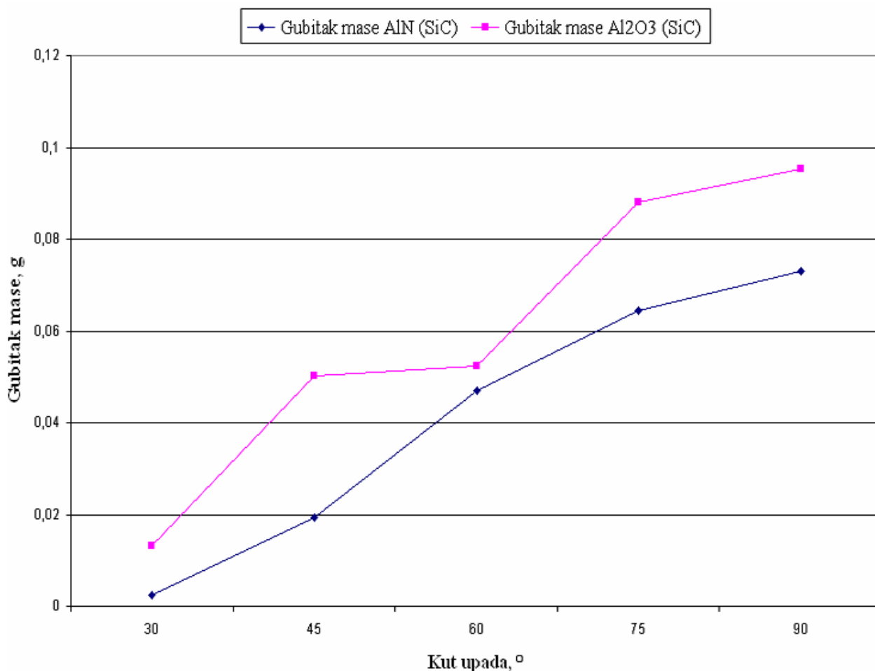
Slika 27. Dijagramski prikaz gubitaka mase ispitanih vrsta keramike, erodiranih silicij karbidnim pijeskom, u ovisnosti o kutu udara čestica
