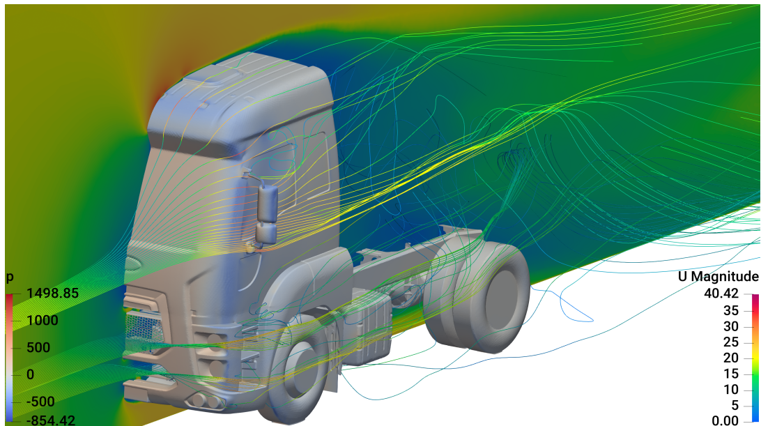
Slika 15: Ford Otosan kamion, izotermno strujanje: aerodinamika.
