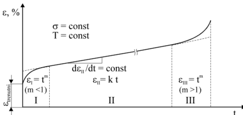
Slika 4. Dijagram puzanja [5]
